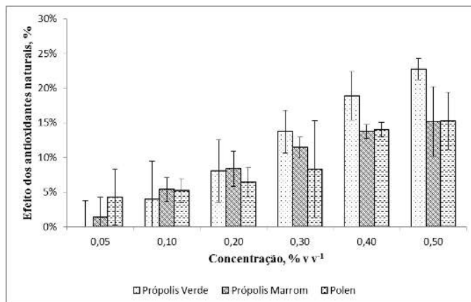
Figura 1. Comparação dos efeitos dos antioxidantes naturais no biodiesel metílico de soja.
